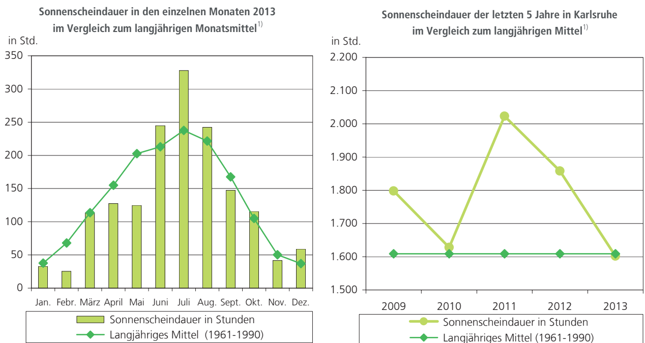
ABBILDUNG 6.4: DIE SONNENSCHENDAUER IN KARLSRUHE IM VERGLEICH ZUM LANGJÄHRIGEN MITTEL 1) (JAHRESSUMME: 1.609 STUNDEN)
